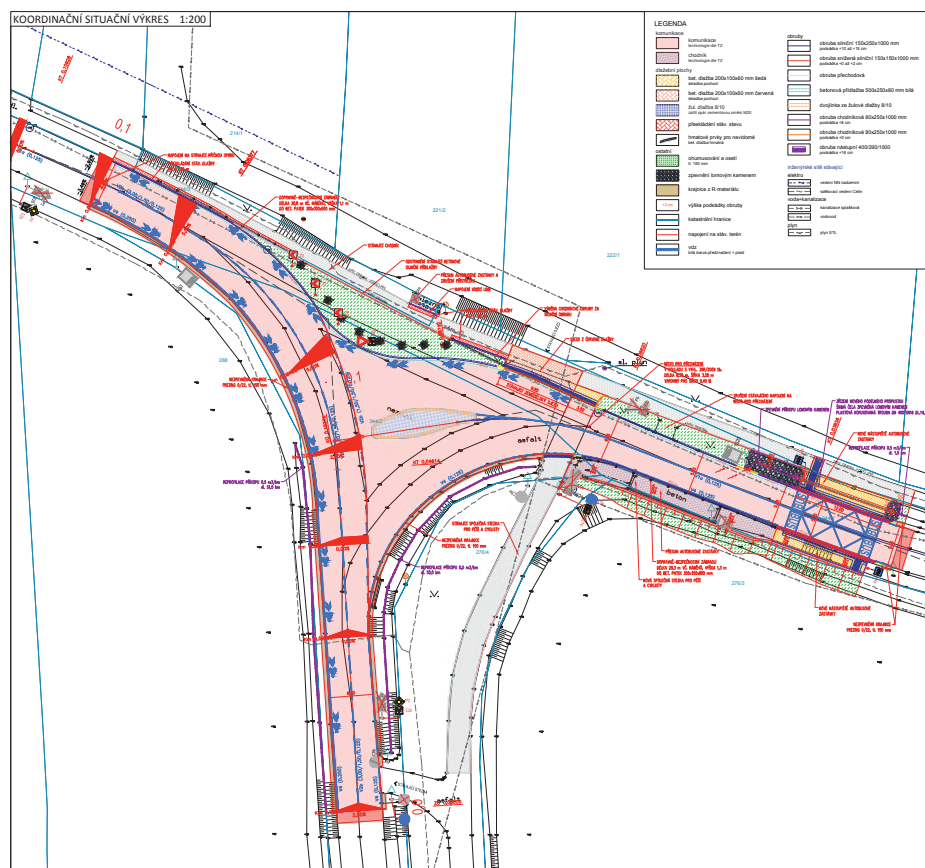
Situace nového uspořádání křižovatky v Hrádku, zdroj: SÚS Pk
